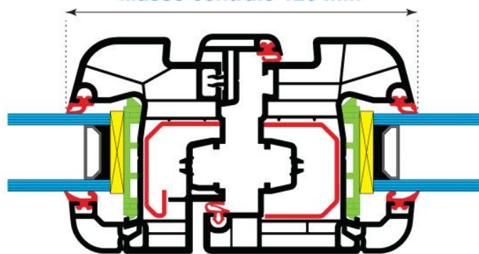
OUVRANT SEMI AFFLEURENT / 6 chambres Masse centrale 126 mm
