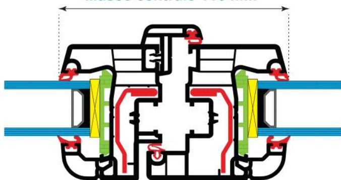
OUVRANT PLAT / 4 chambres Masse centrale 116 mm
