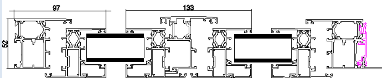
Montage châssis 2 vantaux
