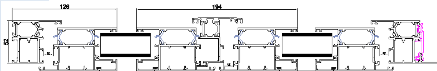
Montage Porte Fenêtre 2 Vantaux
