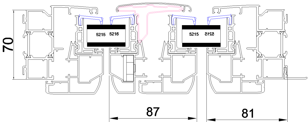
Fenêtre 2 vantaux
