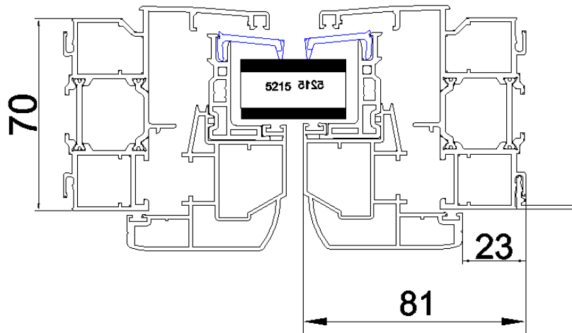
Fenêtre 1 vantail
